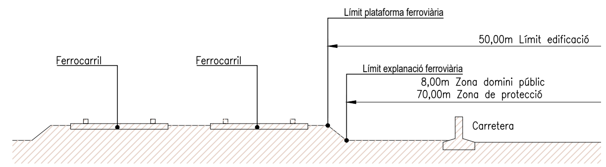
SECCIÓ ESQUEMÀTICA SERVITUDS FERROVIÀRIES Esc. 1:100
