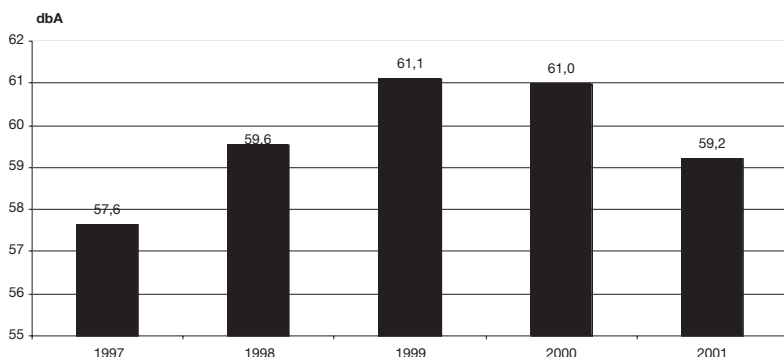
GRÀFIC 107. Evolució dels sorolls de major freqüència (Leq10). Mataró. 1997 - 2001
