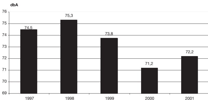
GRÀFIC 105. Evolució de l'indicador de nivell sonor equivalent (Leq) Mataró. 1997 - 2001
